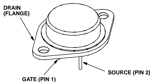
JEDEC TO-204AE
