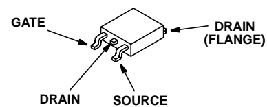
JEDEC TO-252AA
