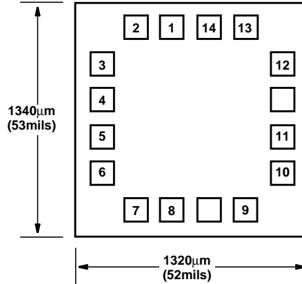
HFA3046
