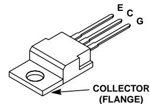
JEDEC TO-220AB
